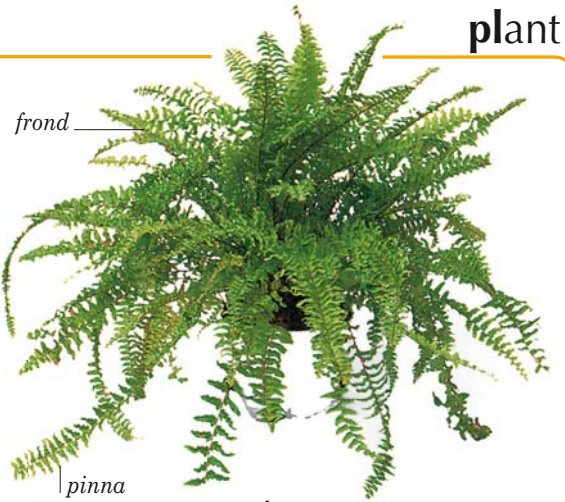
fern
